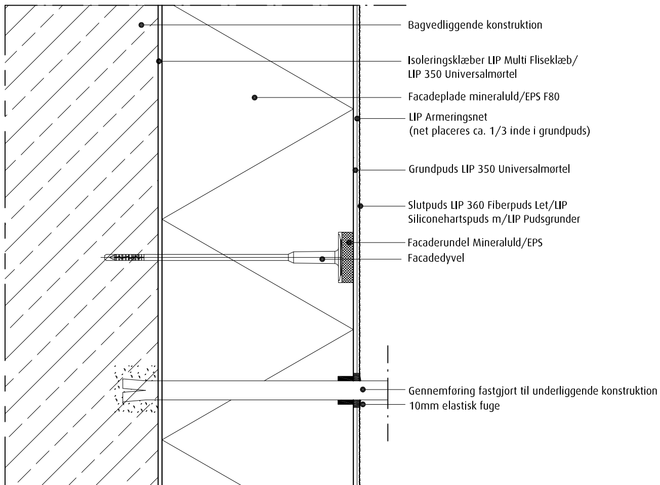
Gennemføring med mekanisk fastgørelse i underliggende konstruktion
