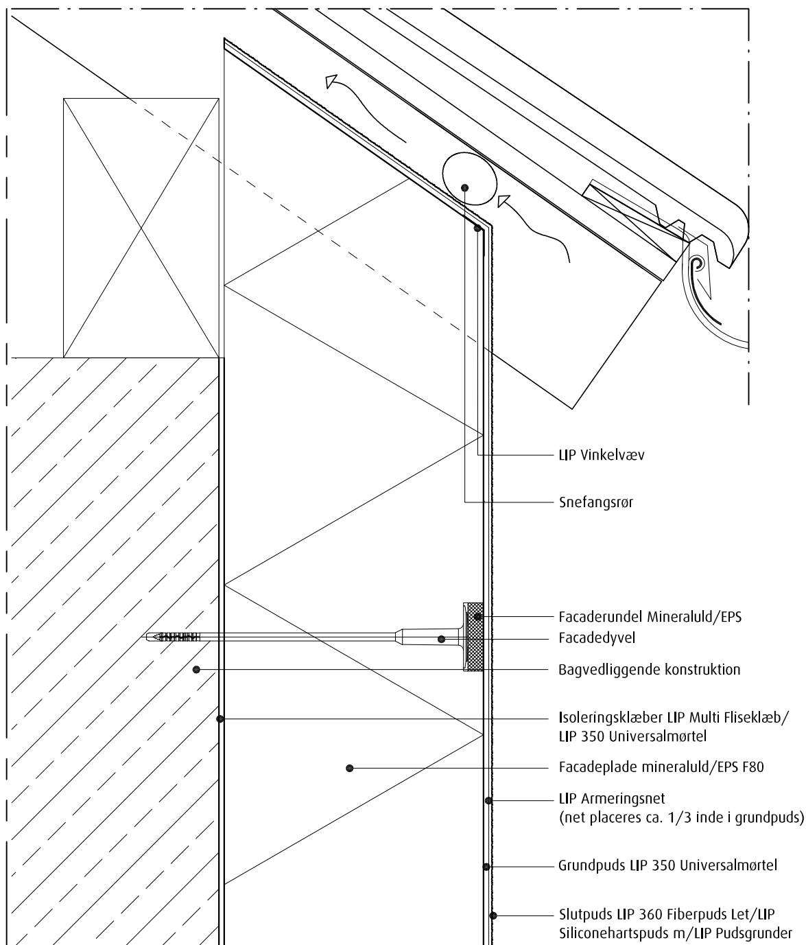
Afslutning ved ventileret tag
