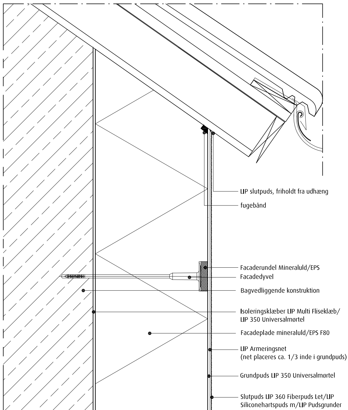
Afslutning ved uventileret tag
