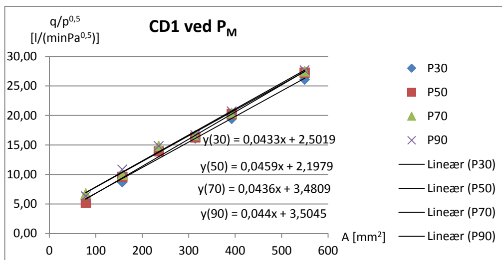
Figur 6 Prøvningsresultater: Relativ luftstrøm ved forskellige tryk q/p^{0,5} for forskellige blændeåbninger A etableret i membranens overside.
