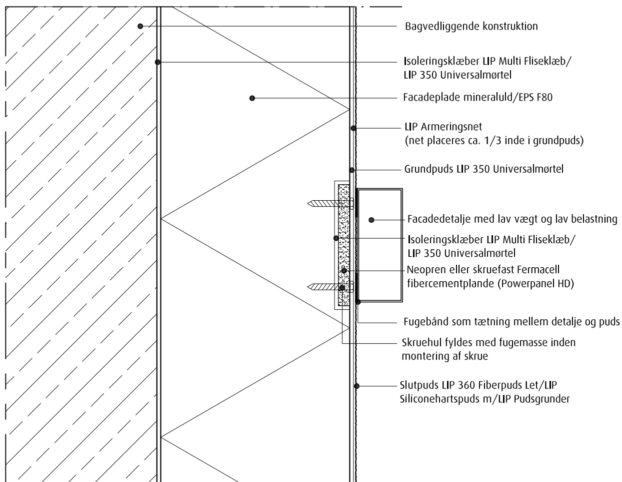
Indfæstning i forstærkningsplade
